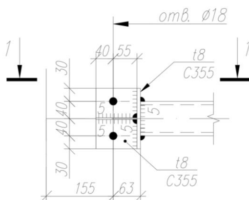
Рис. 1.3.1 Фасонка связи.
