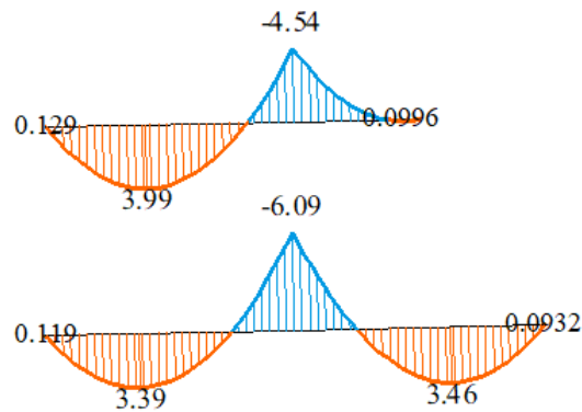
РСН1(СП 20.13330.2011/2016_1) Эпюра Му Единицы измерения - т*м
