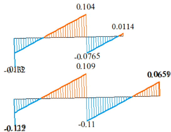
РСН2(СП 20.13330.2011/2016_1) Этюра N Единицы измерения - т
