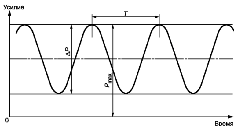
Рисунок Е.1 — Обозначения параметров повторяющейся нагрузки
